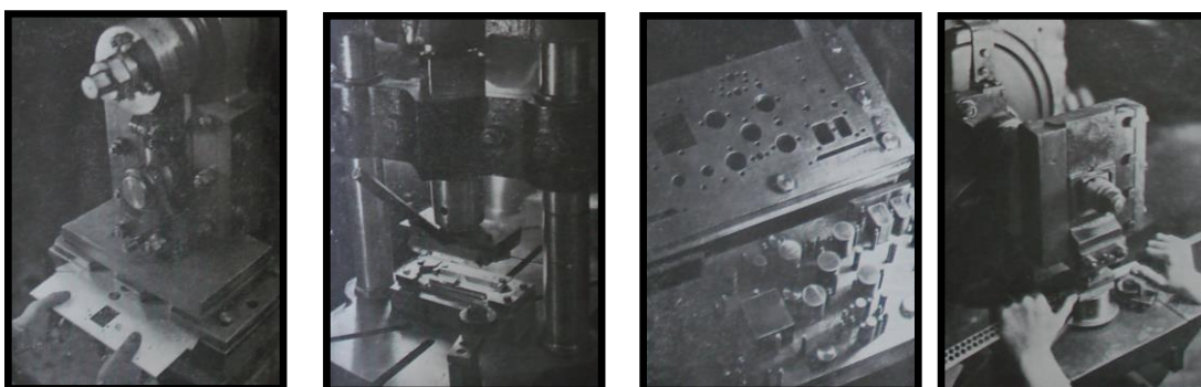
Van links naar rechts: perçage du châssis, emboutissage par une presse de 100 tonnes, découpage (La Radio-Industrie, Bruxelles, 1934).
