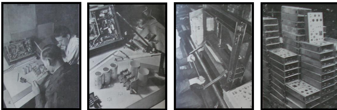
Van links naar rechts: het productieproces van omroepontvangers bij F.N.R.: la conception, vers la réalisation, pliage du châssis, châssis (La Radio-Industrie, Bruxelles, 1934).
