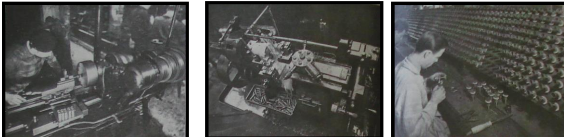
Van links naar rechts: tours de décolletage automatiques, achèvement des bobinages (La Radio-Industrie, Bruxelles, 1934)
