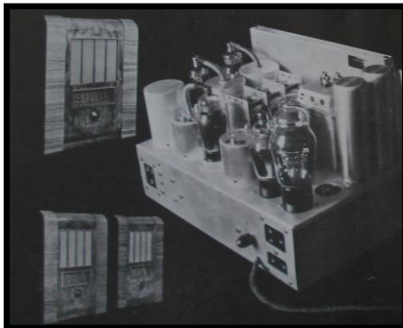
Links: het afgewerkte product (La Radio-Industrie, Bruxelles, 1934)
